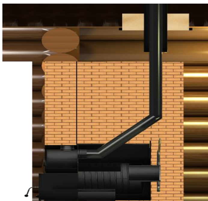
Рис.4 Установка печи
